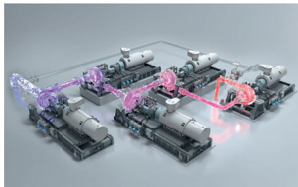
性能数据：用于蒸汽再压缩的串联系统
